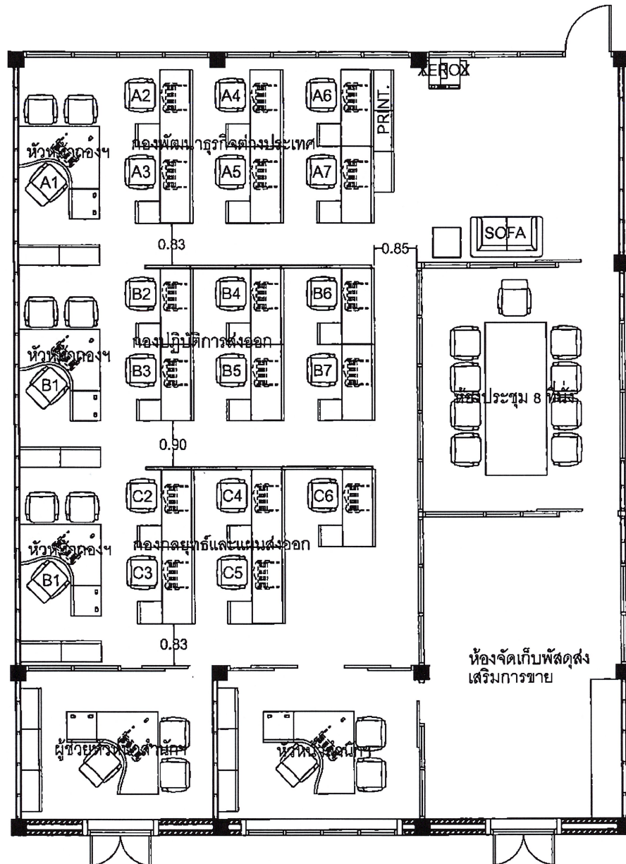
ห้องทำงานสำนักส่งออกและตลาดต่างประเทศ มาตราส่วน 1 : 100
