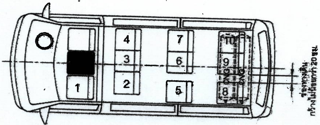
รถตู้โดยสารที่ใช้ก๊าซเป็นเชื้อเพลิง
