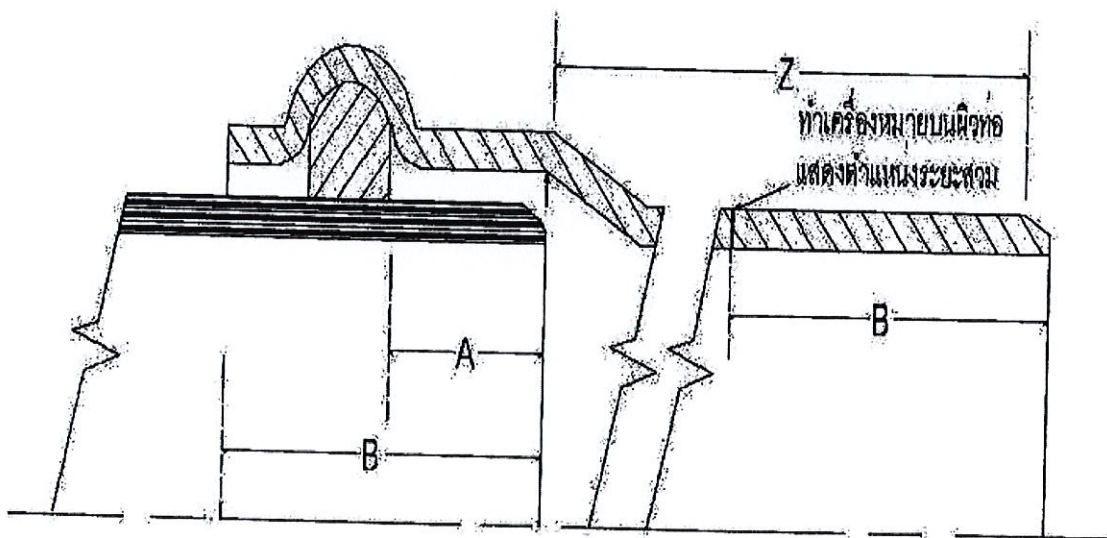
รูปที่ 1 ระยะความลึกของหัวสวม “A” และความยาวใช้งาน
